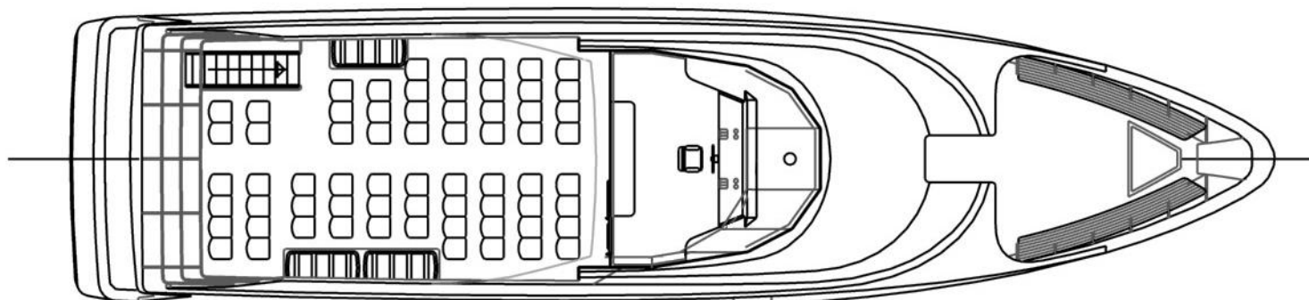
PIANTA PONTE BELVEDERE
